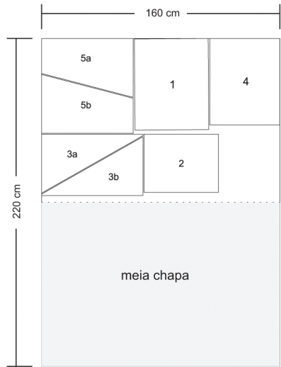
Plano de corte para chapa compensado 15mm
